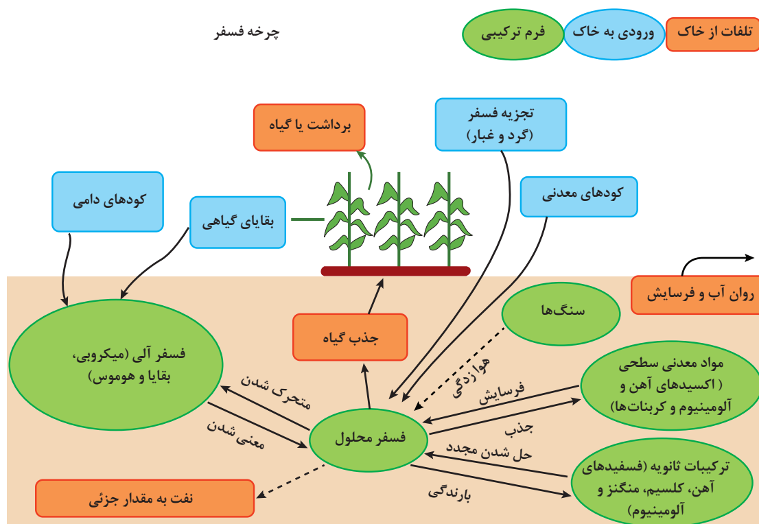
شکل ۱۶- چرخه فسفر
