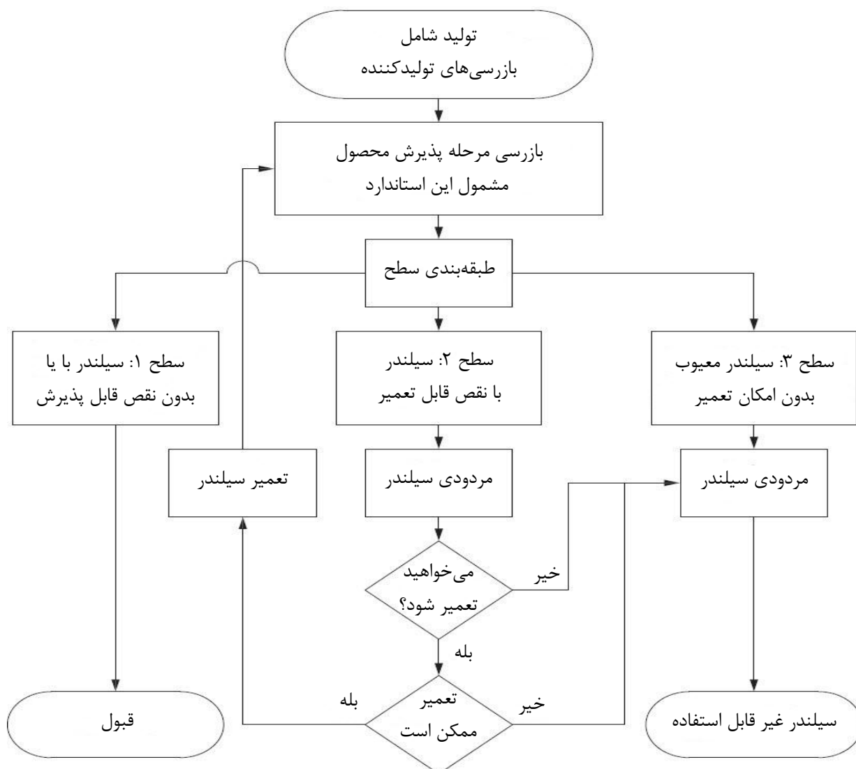
شکل الف-۱- روندنمایی برای بازرسی چشمی نهایی سیلندرهای گاز در زمان پذیرش محصول
