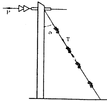
شکل (۱۱) مهار ساده
