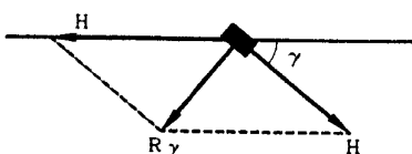
شکل (۶) مؤلفه افقی براینده نیروهای کشش سیم
