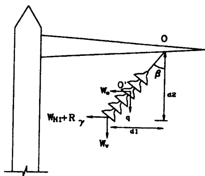
شکل (۸) محاسبه زاویه انحراف مقره
