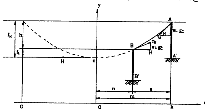
شکل (۹) نیروی بالا برنده
