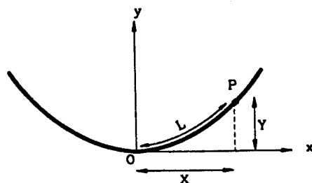
شکل (۲) منحنی سیم
