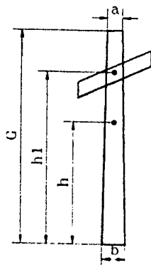
شکل (۷) فواصل مختلف روی پایه
