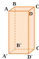
منشور چهارپهلوی
