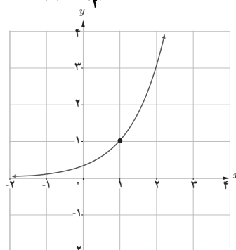
(۵) j(x) = 3^{(x-1)} ث)
