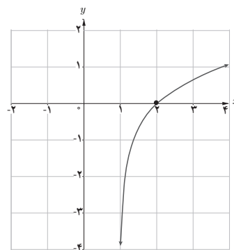
(۲) g(x) = \log(x-1) ت)
