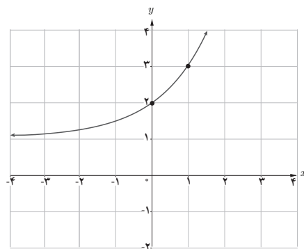
(۱) f(x) = 2^x + 1 ج)
