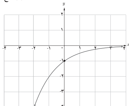
(۳) h(x) = -\left(\frac{1}{2}\right)^x پ)
