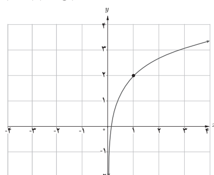
(۴) l(x) = 2 + \log x ب)
