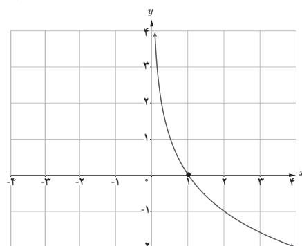
(۶) k(x) = -\log_2 x الف)
