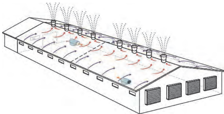
تهویه سقفی
