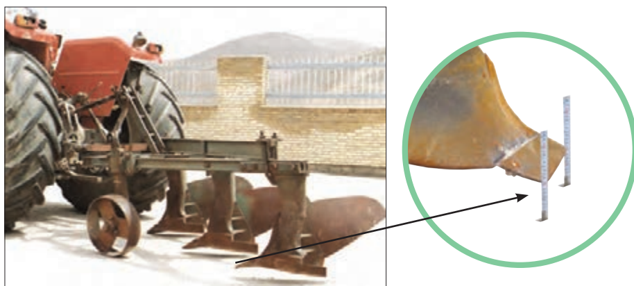
شکل ۳۱- تنظیم تراز عرضی گاواهن
