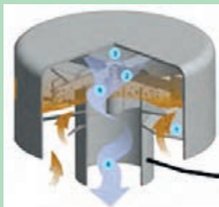
شکل ۱-۲۵ اصول کار پیش صافی
