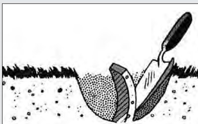
شکل ۱۴-۲- روش برداشت نمونه با بیل یا بیلچه
