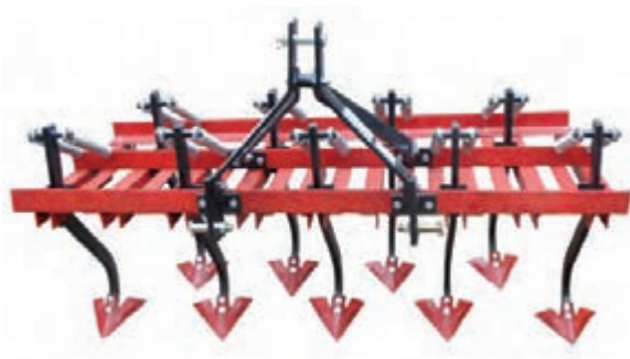
شکل ۴-۱۰- کولتیواتور با تیغه پنجه غازی
