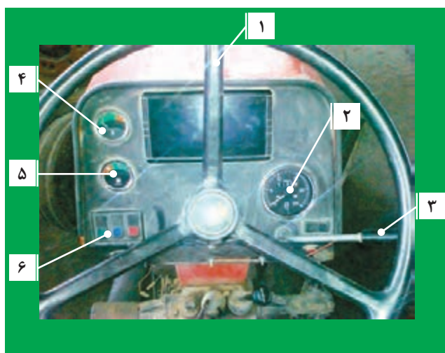
شکل ۱-۶- تجهیزات کنترلی تراکتور MF۲۸۵
