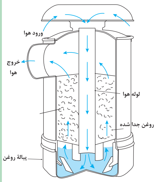
شکل ۱-۲۷ اصول کار صافی روغنی
