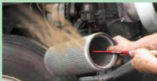
شکل ۳۵-۱- تمیز کردن صافی خشک با فشار هوا
