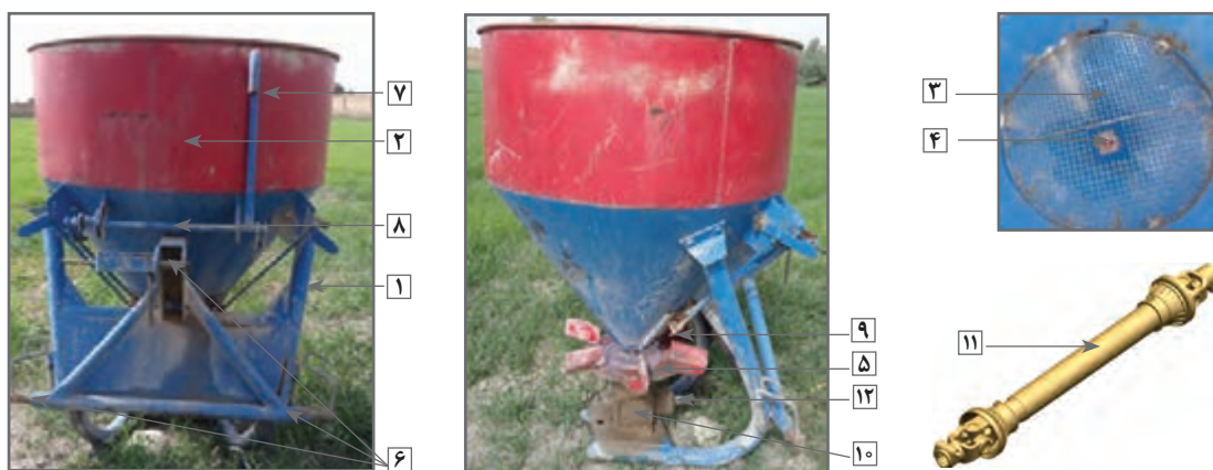
شکل ۷- قسمت‌های مختلف بذریاش سانتریفیوژ
