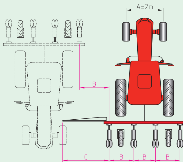
شکل ۲۲- تنظیم علامت‌گذار
