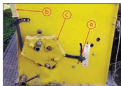
شکل ۸ a: درجه ریزش بذر (تغییر سرعت موزع) b: اهرم تنظیم ریزش بذر (دریچه زیر موزع) c: جعبه دنده
