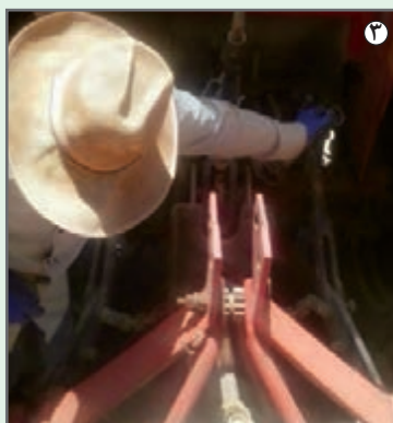
شکل ۴۸- ابتدا اتصال بازوی چپ سپس بازوی سمت راست، چهارشاخ گاردان و نهایتاً بازوی وسط
