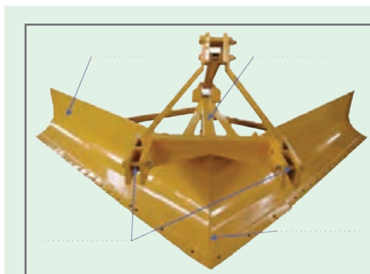
شکل ۲۱- ساختمان نهركن
