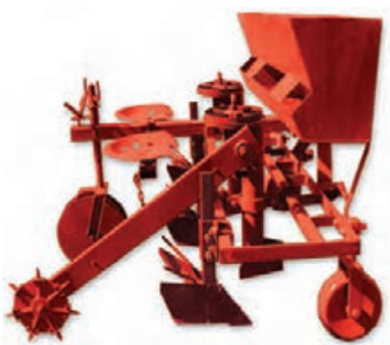
شکل ۳- غده کار نیمه خودکار متداول با موزع افقی
