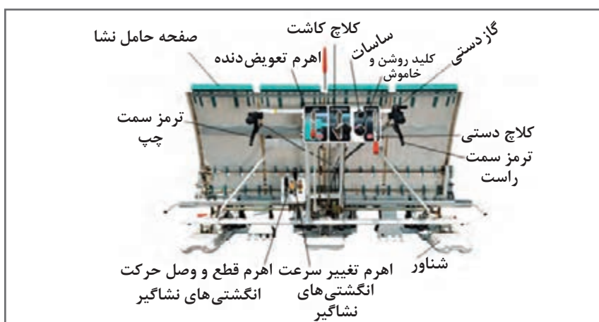
شکل ۱۰- اجزای نشاکار راهرونده از نمای پشت
