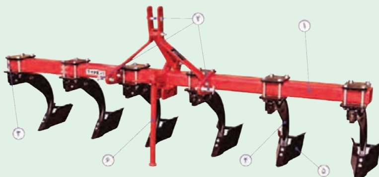
شکل ۱۳- ساختمان شیارکش
