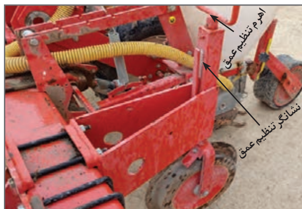
شکل ۱۸- تنظیم عمق کاشت
