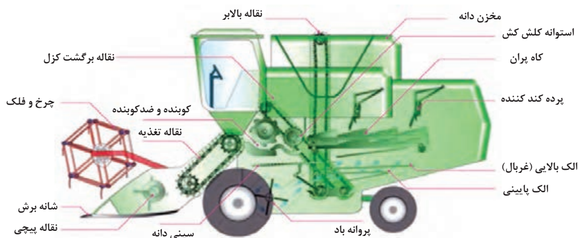
شکل ۳- کمباین غلات
