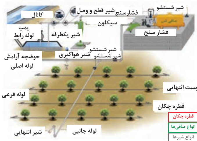
شکل ۱۵- اجزای سیستم آبیاری قطره‌ای
