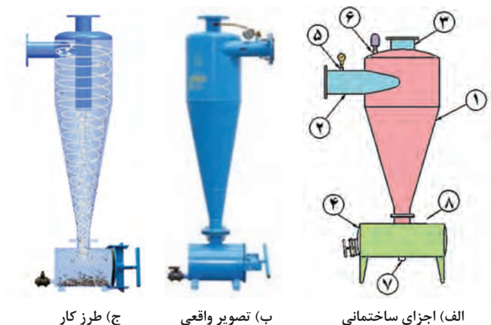
شکل ۲۱- هیدروسیکلون
