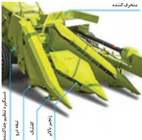
شکل ۴۷- دماغه چابر دو ردیفه کششی
