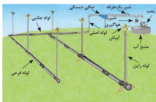
شکل ۷- شبکه آبیاری بارانی کلاسیک
