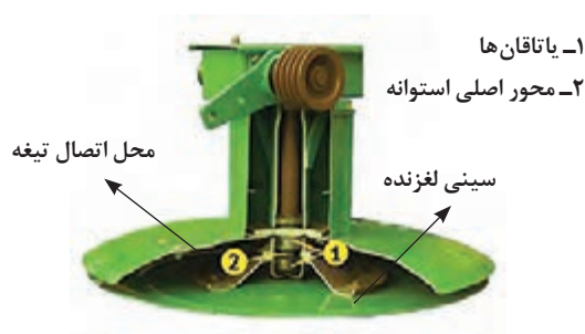
شکل ۴- شماتیک داخلی جعبه دنده و محور اصلی استوانه‌ها و سینی زیر دروگر استوانه‌ای
