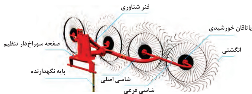
شکل ۳- ردیف ساز شانه خورشیدی (چرخه)
