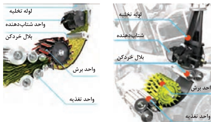
الف) موقعیت واحدهای روی ماشین ب) حرکت علوفه در واحدهای ماشین
