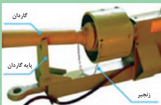
شکل ۶۹- اتصال گاردان به چاپر و مهار پوسته و شیلنگ
