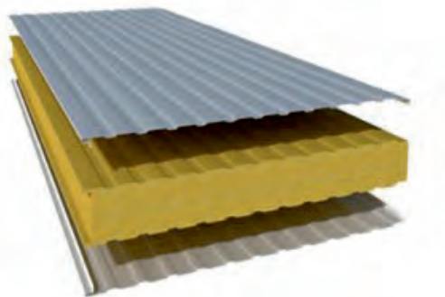
ساندویچ پانل
