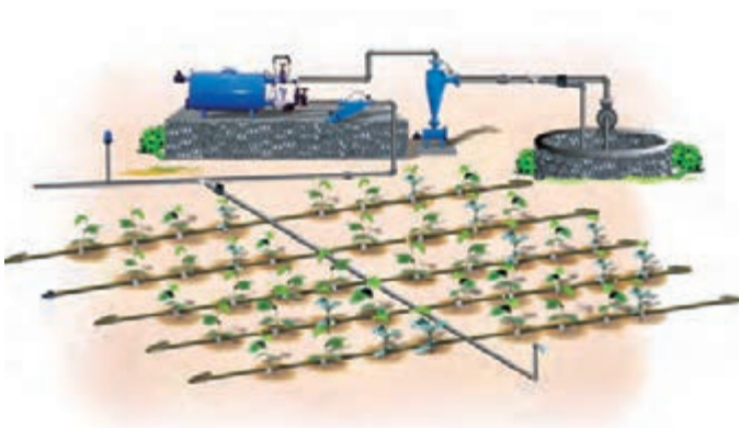
سیستم آبیاری قطره‌ای
