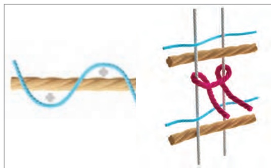
الف) نمای روبه‌رو ب) نمای بالا شکل ۴-۲- وضعیت قرارگیری تار و پودها در شیوه نیم لول
