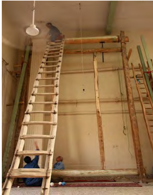
شکل ۲۱-۱ دار ثابت چوبی برای بافت قالی و گلیم
