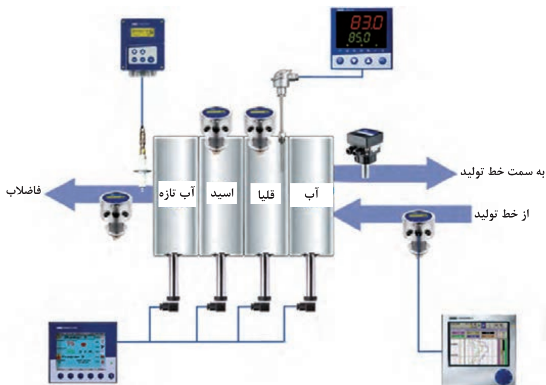
شکل ۱-۲۲- سیستم CIP
