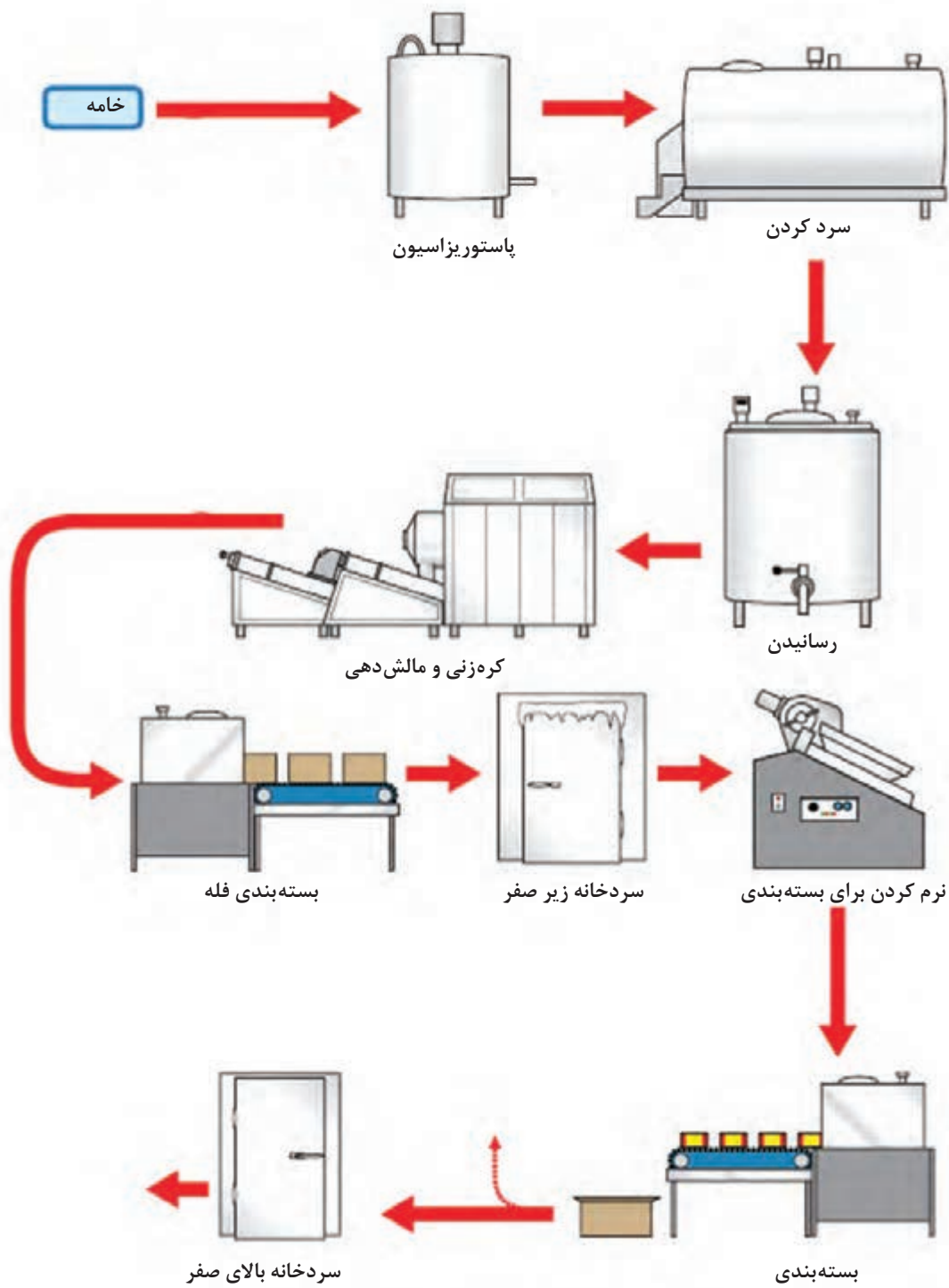
شکل ۱۱-۵- فرایند تولید کره
