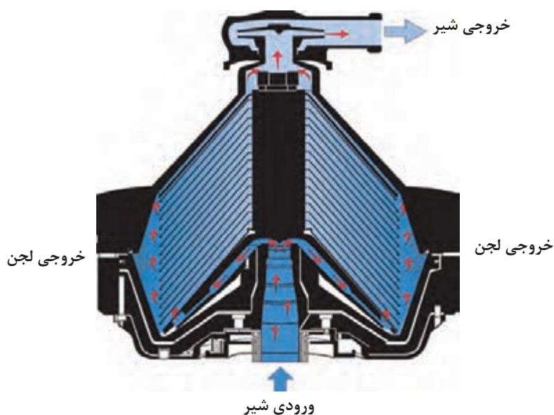
شکل ۱-۱۰ کلاریفایر
