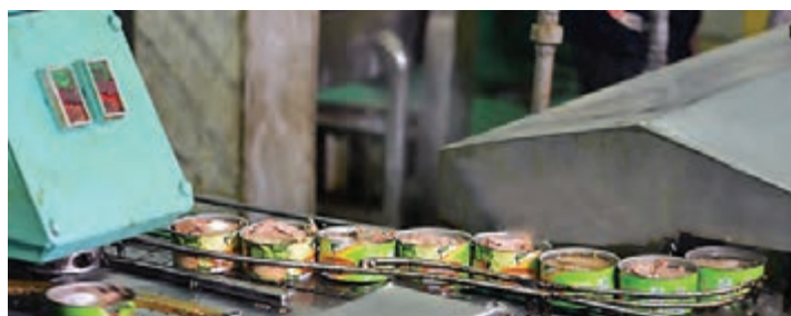
شکل ۲- ورود به تونل بخار
