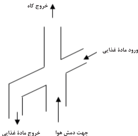
شکل ۱- اصول کار آسپیراتور
