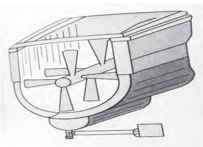
شکل ۶- مقطع مخلوط کن یک شافتی مجهز به سیستم جریان آب
