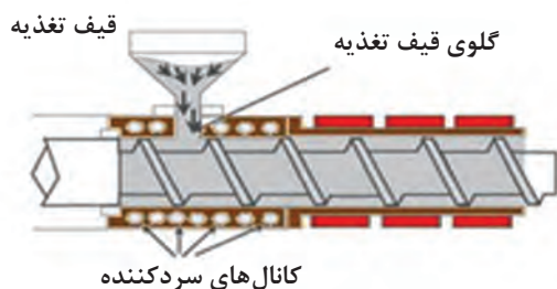
شکل ۹- اکسترودر
