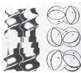
شکل ۸- نحوه ورزیدن خمیر ماکارونی در مارپیچ دو گانه
