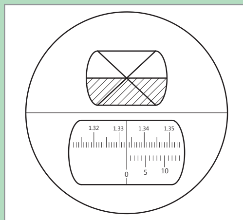
شکل ۱۱- صفحه تنظیم رفراکتومتر روغن
