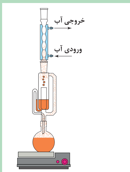
شکل ۷- دستگاه سوکسله
