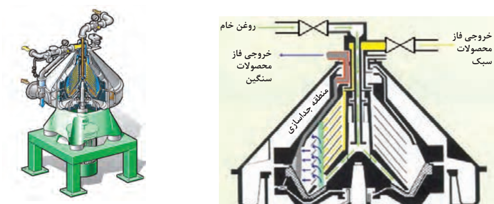
شکل ۷- شماتیک سانتریفیوژ
