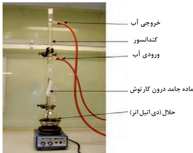
شکل ۳- دستگاه سوکسله
