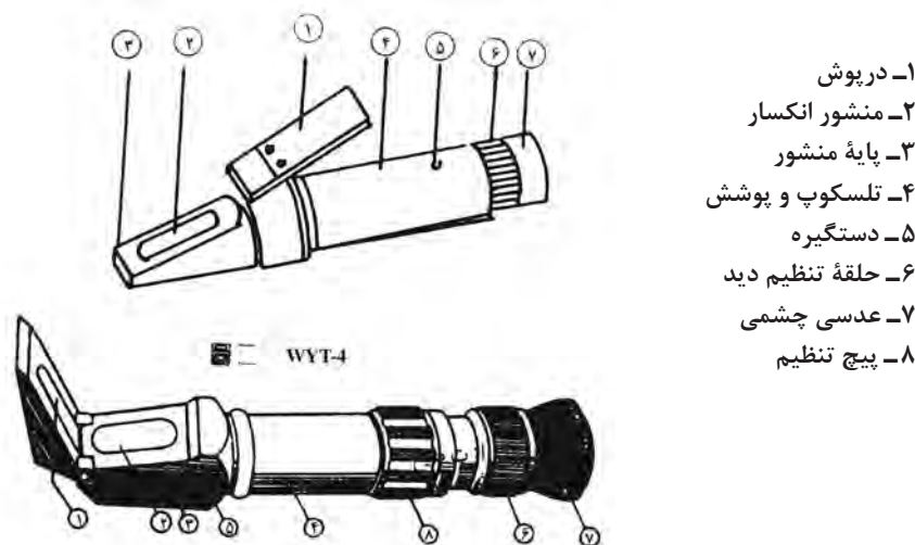
شکل ۳- رفاکتومترهای دستی
