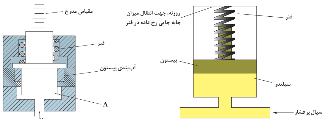
شکل ۱۴- مانومتر نوع پیستونی
