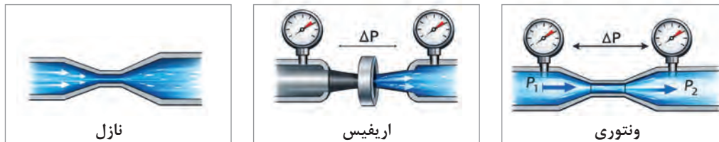
شکل ۱۰- وسایل اندازه‌گیری جریان سیالات
