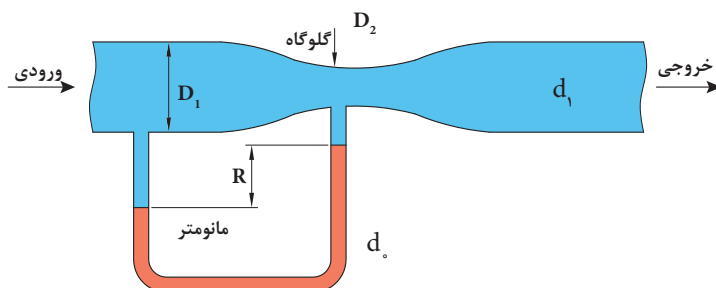
شکل ۱۵- ونتوری متر با مانومتر دیفرانسیلی
