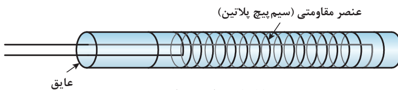
شکل ۱۵- دماسنج مقاومتی
