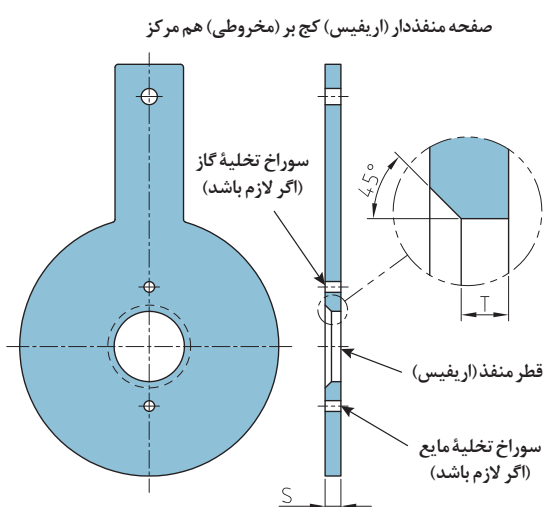
شکل ۱۲- طرح ساده‌ای از روبه‌رو و پهلوی اریفیس متر
