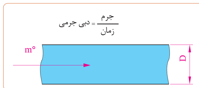
شکل ۲- نمایشی از دبی جرمی در خط لوله ( m^\circ : دبی جرمی سیال و D: قطر خط لوله)
