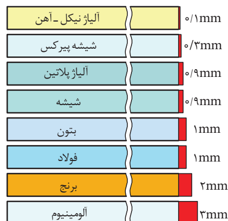
شکل ۱۶- میزان انبساط یک متر از اجسام مختلف در اثر افزایش دمای ۱۰۰ درجه سلسیوس
