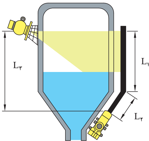
شکل ۱۶- سطح‌سنج رادیواکتیو
