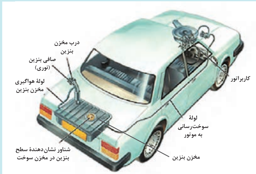
جایگاه مخزن بنزین در خودرو
