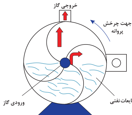
شکل ۱۹- نمای درونی جریان سنج گاز به روش تر
