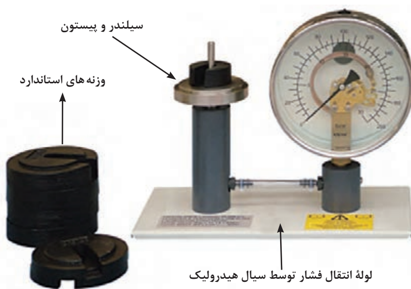
شکل ۱۹- سامانه تنظیم فشارسنج بوردون به روش بار مرده
