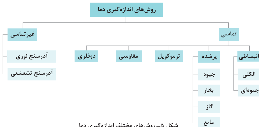
شکل ۵- روش‌های مختلف اندازه‌گیری دما
