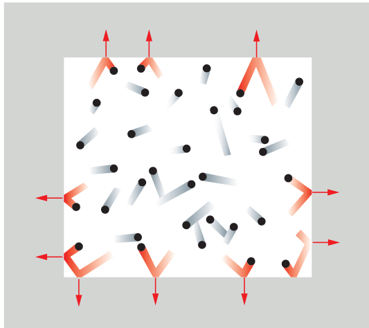
شکل ۲ - نمایش حرکت مولکول‌ها در گازها
