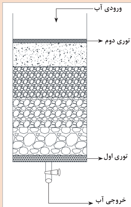
شکل ساده‌ای از صافی شنی
