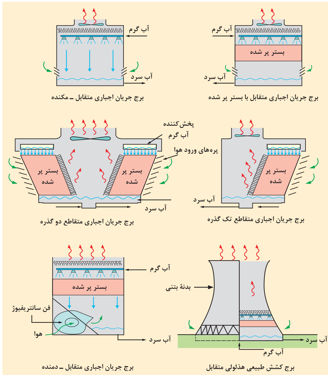
شکل ۱۱- انواع آرایش‌های برج‌های خنک‌کننده مرطوب
