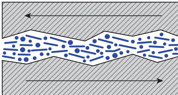
شکل ۱۱- شیوه عملکرد روانکار جامد
