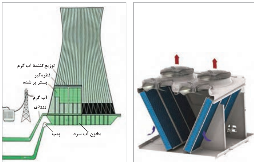
شکل ۱۲- طرح ساده ای از یک برج خنک کننده خشک
