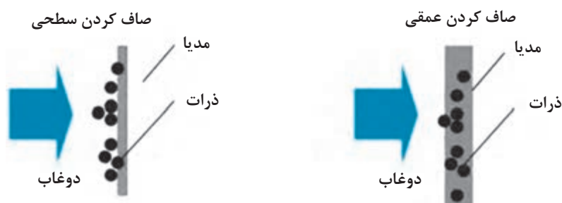
شکل ۶- انواع فیلتراسیون (بر حسب چگونگی حرکت سیال)
