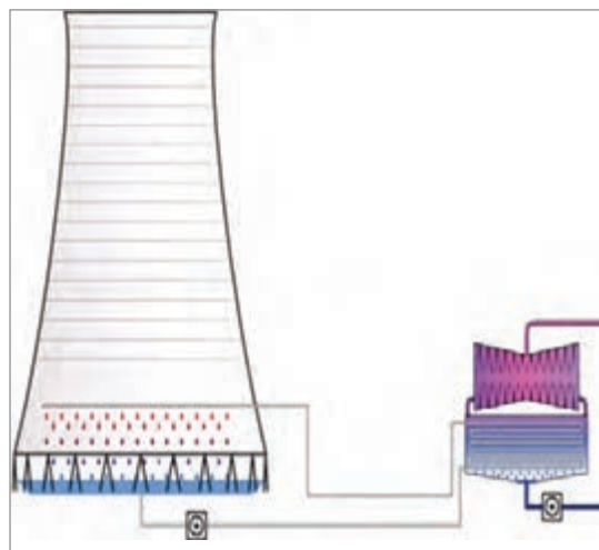
شکل ۱۳- طرح ساده‌ای از یک برج خنک‌کننده خشک-مرطوب
