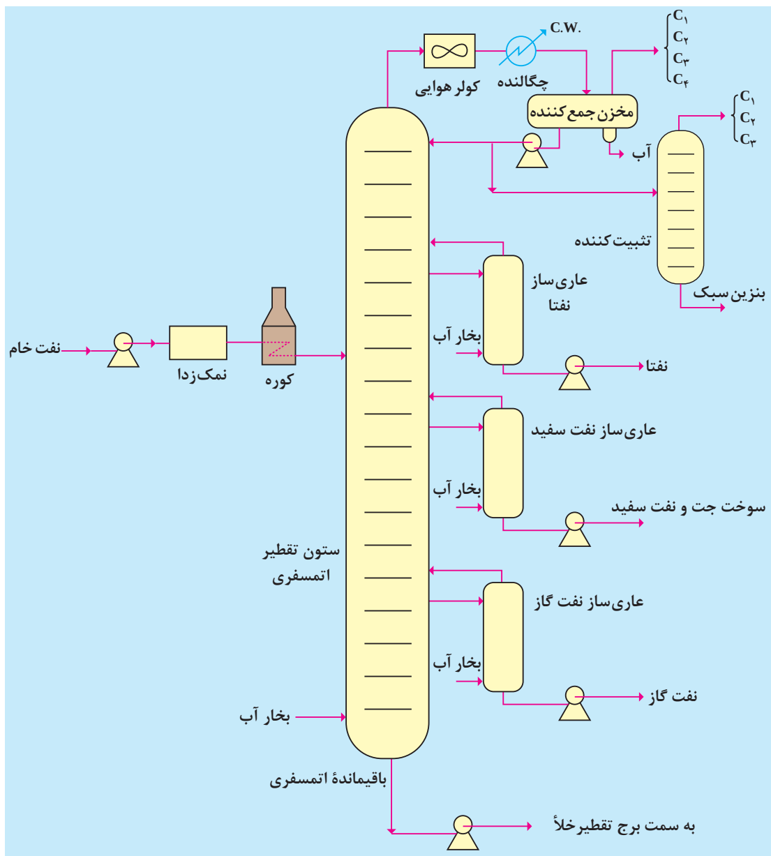
شکل ۶- تقطیر اتمسفری نفت خام
