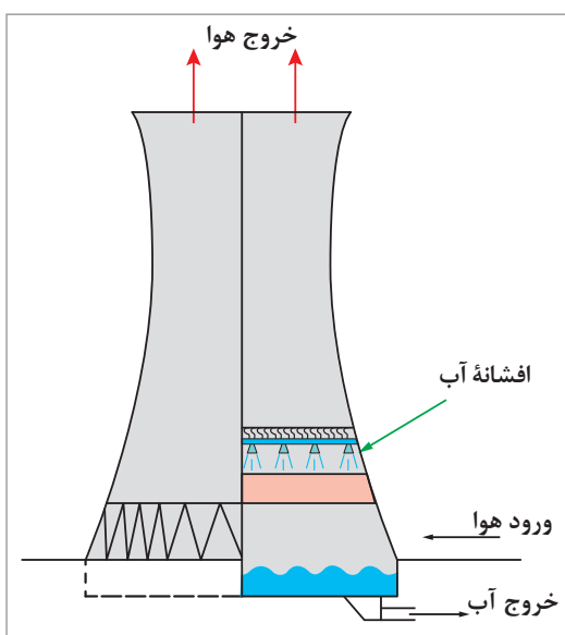
شکل ۹- طرح ساده‌ای از یک برج خنک‌کنندهٔ مرطوب
