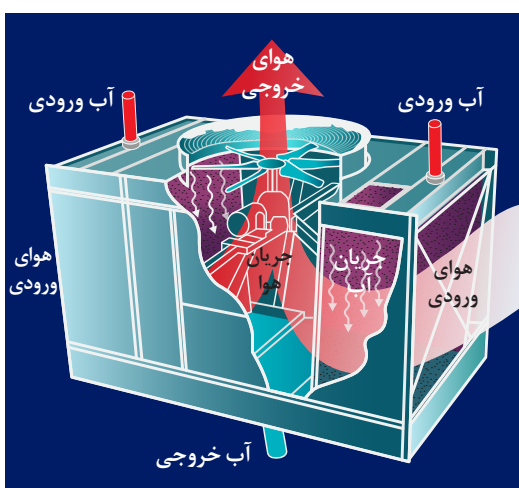
شکل ۱۰- نمایی برش خورده از برج خنک‌کنندهٔ مرطوب
