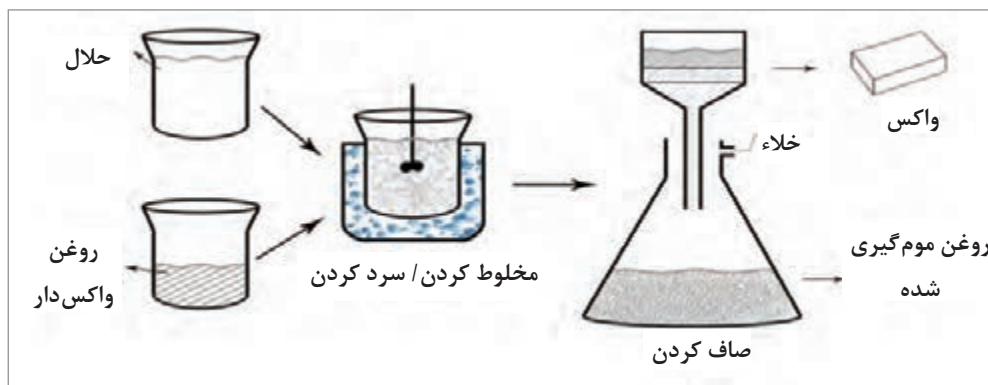
شکل ۸- جداسازی موم از روغن
