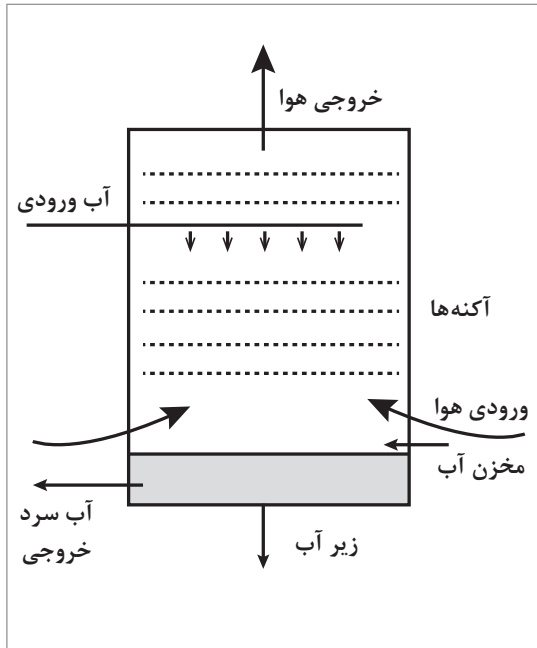
شکل ۷- طرح ساده‌ای از نمای داخلی و خارجی یک نمونه برج خنک‌کننده آزمایشگاهی
