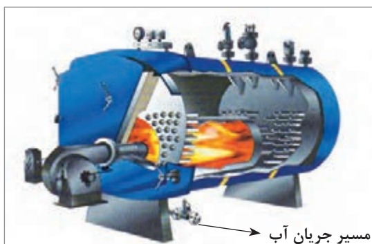
شکل ۷- تصویر واقعی و نمای داخلی زیر آبکشی از یک نوع دیگ بخار
