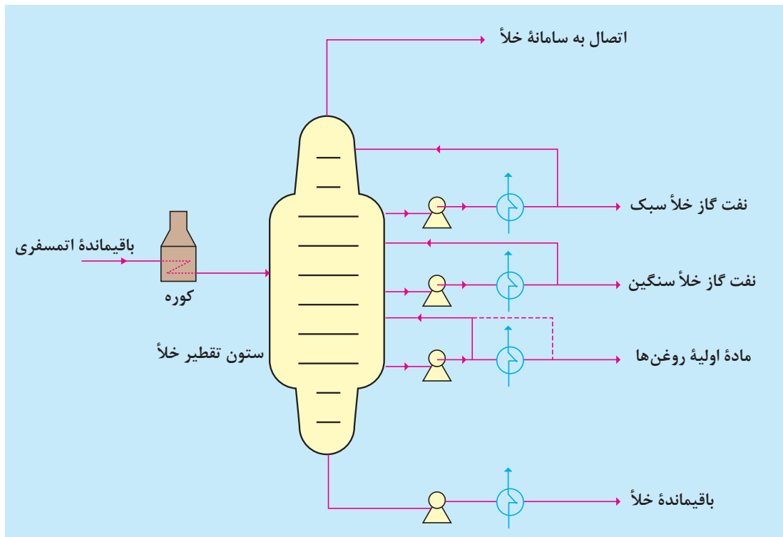
شکل ۷- تقطیر خلأ باقیمانده اتمسفری
