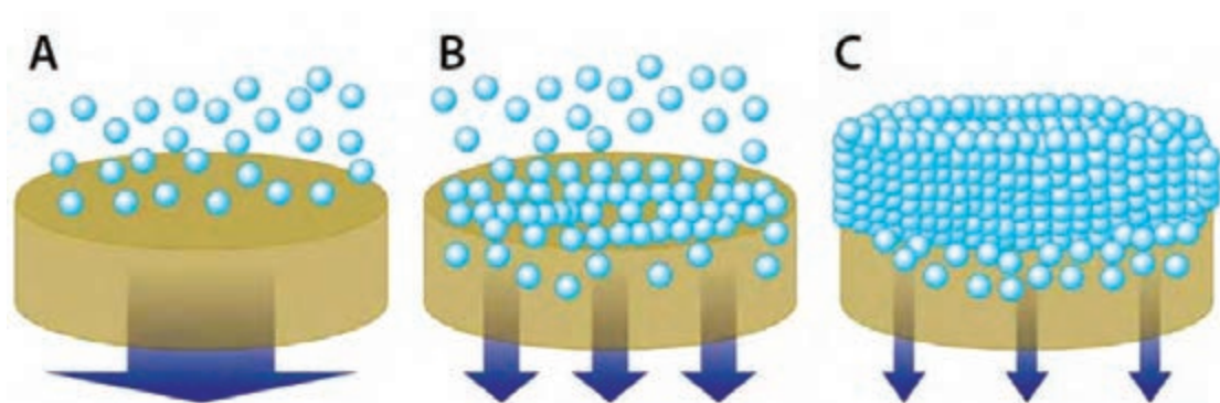
شکل ۲۱- تجمع ذرات جامد بر روی پارچه فیلتر
