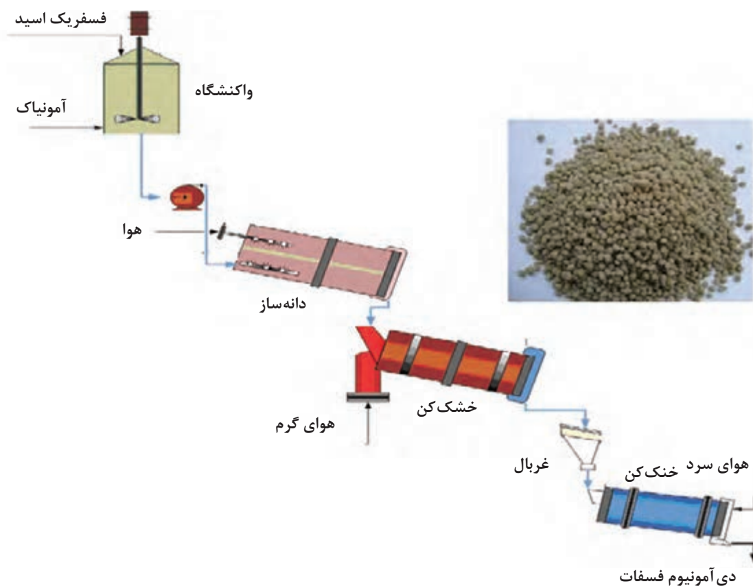
شکل ۹- فرایند تولید دی‌آمونیم فسفات
