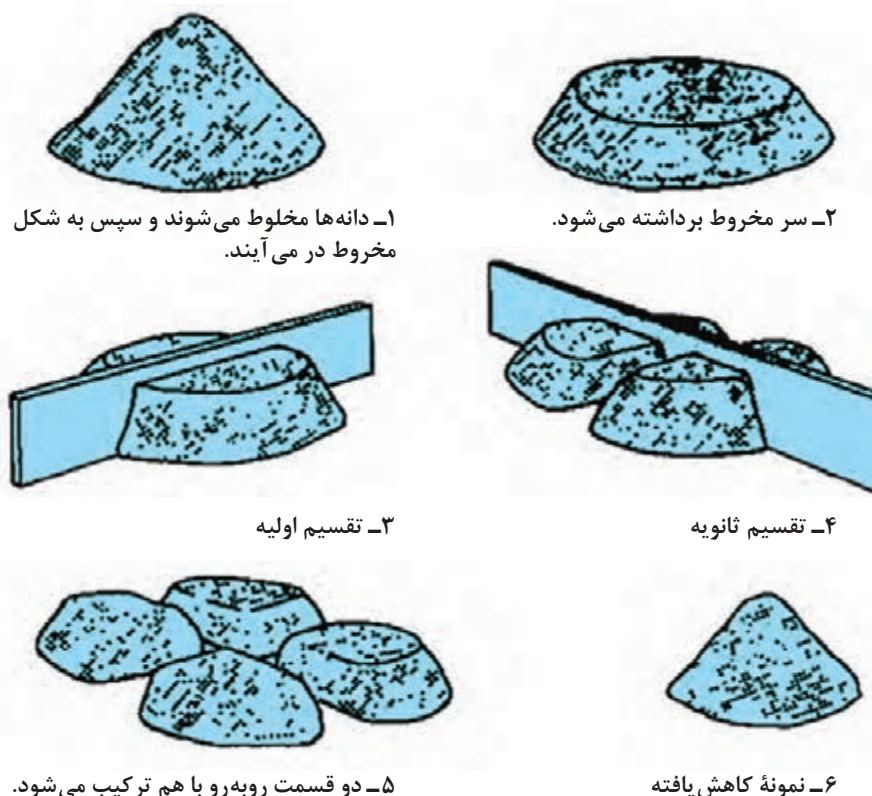
شکل ۱۲- مخروط کردن و سپس یک چهارم کردن
