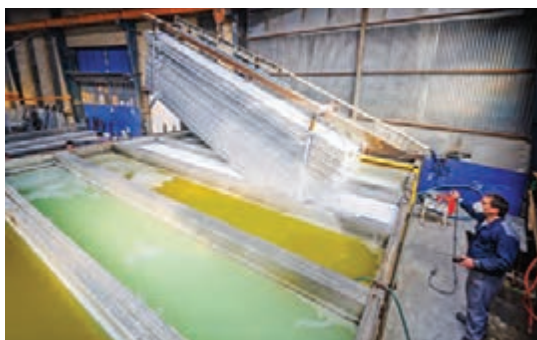
شکل ۸- مخزن آبکاری با میله‌های آندی و کاتدی
