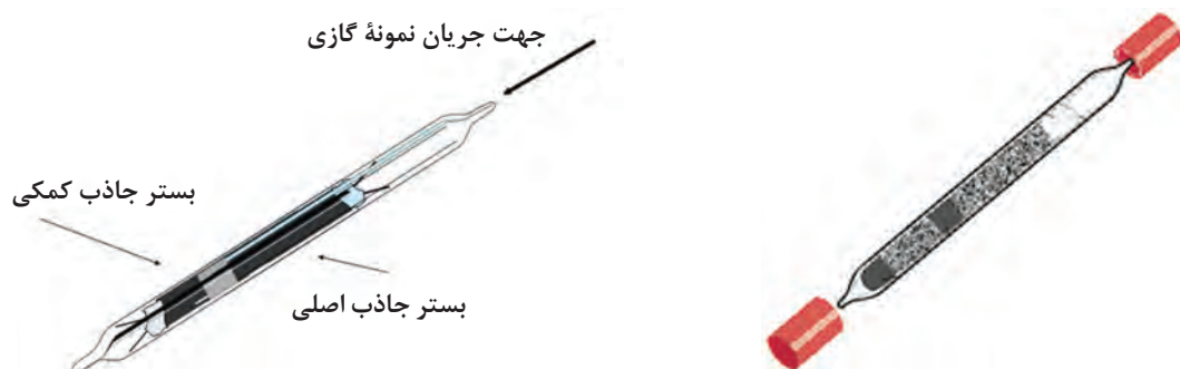
شکل ۲۰- لوله جاذب سطحی حاوی زغال فعال
