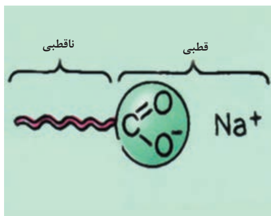
شکل ۱۶- الف) سرهای قطبی و ناقطبی در مولکول ماده فعال کننده سطح
