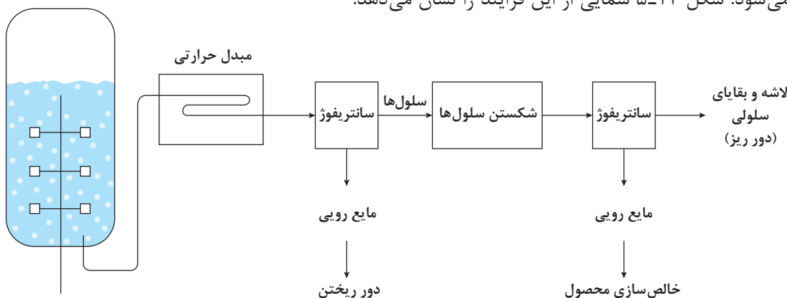
شکل ۵-۱۴- طرح ساده‌ای از فعالیت‌هایی که پس از فرایند تخمیر برای جداسازی آنزیم‌های درون سلولی انجام می‌شود.
