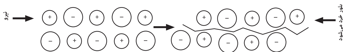
شکل (۳-۴) بر اثر جابه‌جا شدن یک ردیف از یون‌ها، بارهای همانم یکدیگر را دفع می‌کنند و سبب فرو ریختن ساختار بلور می‌شوند.
