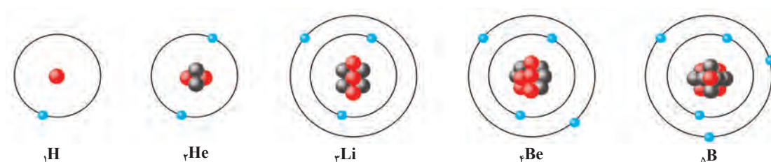
شکل (۲-۵) مدل اتمی بور برای اتم‌های هیدروژن، هلیوم، لیتیم، بریلیم و بور
