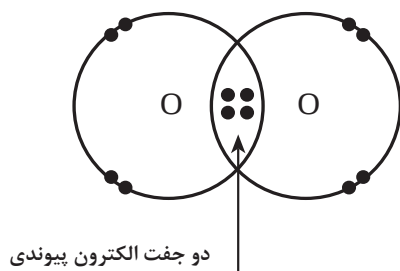
شکل (۳-۸) آرایش الکترونی لایه ظرفیت در مولکول \text{O}_2
