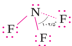
ساختار لوئیس NF_3
