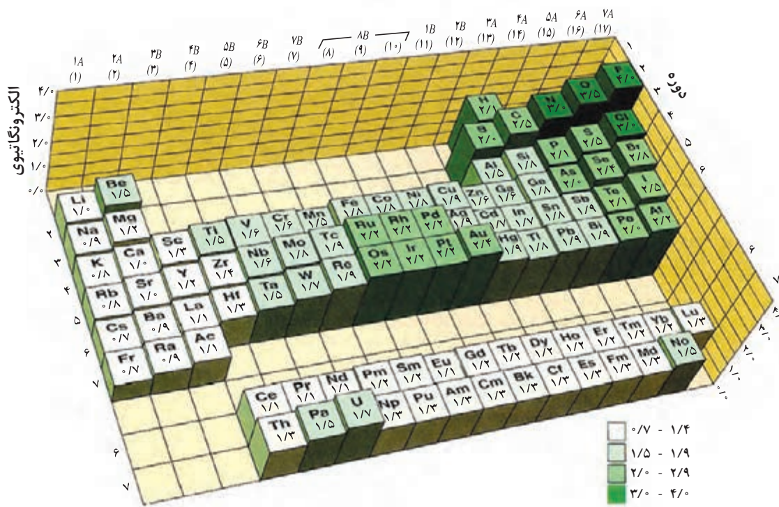
شکل (۳-۱۰) الکترونگاتیوی نسبی عناصر در جدول تناوبی
