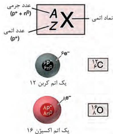
شکل (۲-۲) نماد شیمیایی اتم‌ها
