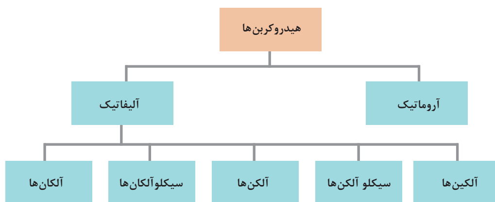
شکل ۱- طبقه‌بندی هیدروکربن‌ها
