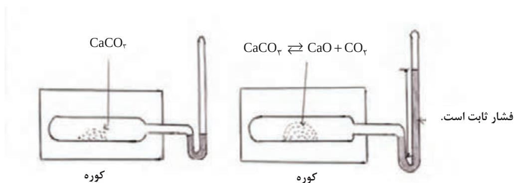
شکل ۱۲- فشار ایجادشده در اثر فرایند تجزیهٔ کلسیم‌کربنات در دمای 1073^\circ\text{K}
