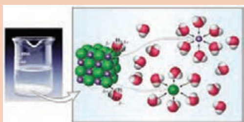
فرایند حل‌شدن نمک طعام در آب
