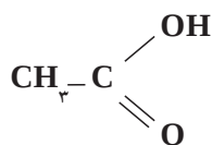
استیک اسید
