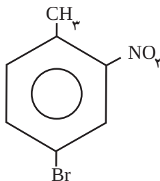
۴- برمو - ۲- نیترو تولوئن
