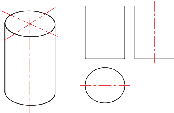
شکل ۵۵- حجم و سه‌نمای استوانه
