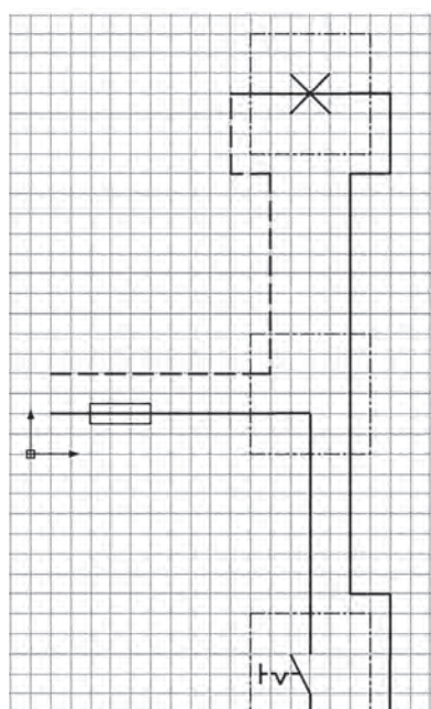
شکل ۲- نقشه حقیقی مدار یک پل
