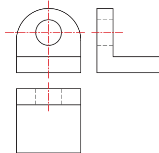
شکل ۵۶- سه‌نما
