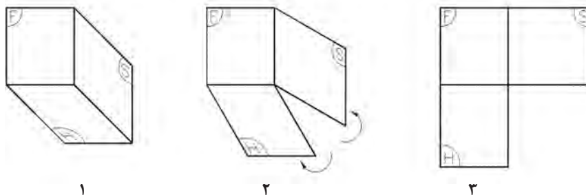
شکل ۲۶- مراحل تسطیح
